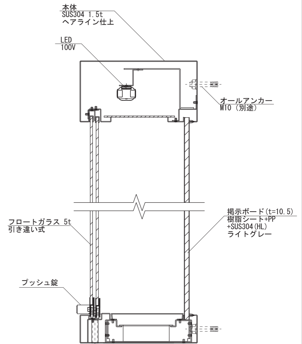
【側断面図 S=1:5】
