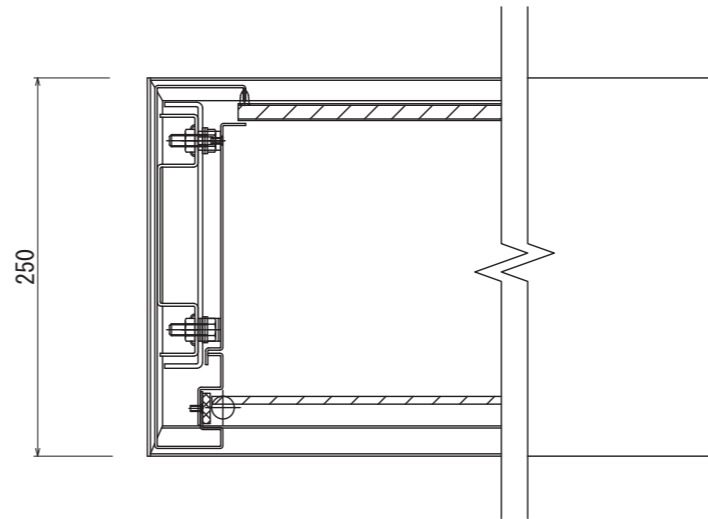
【平面図 S=1:5】
