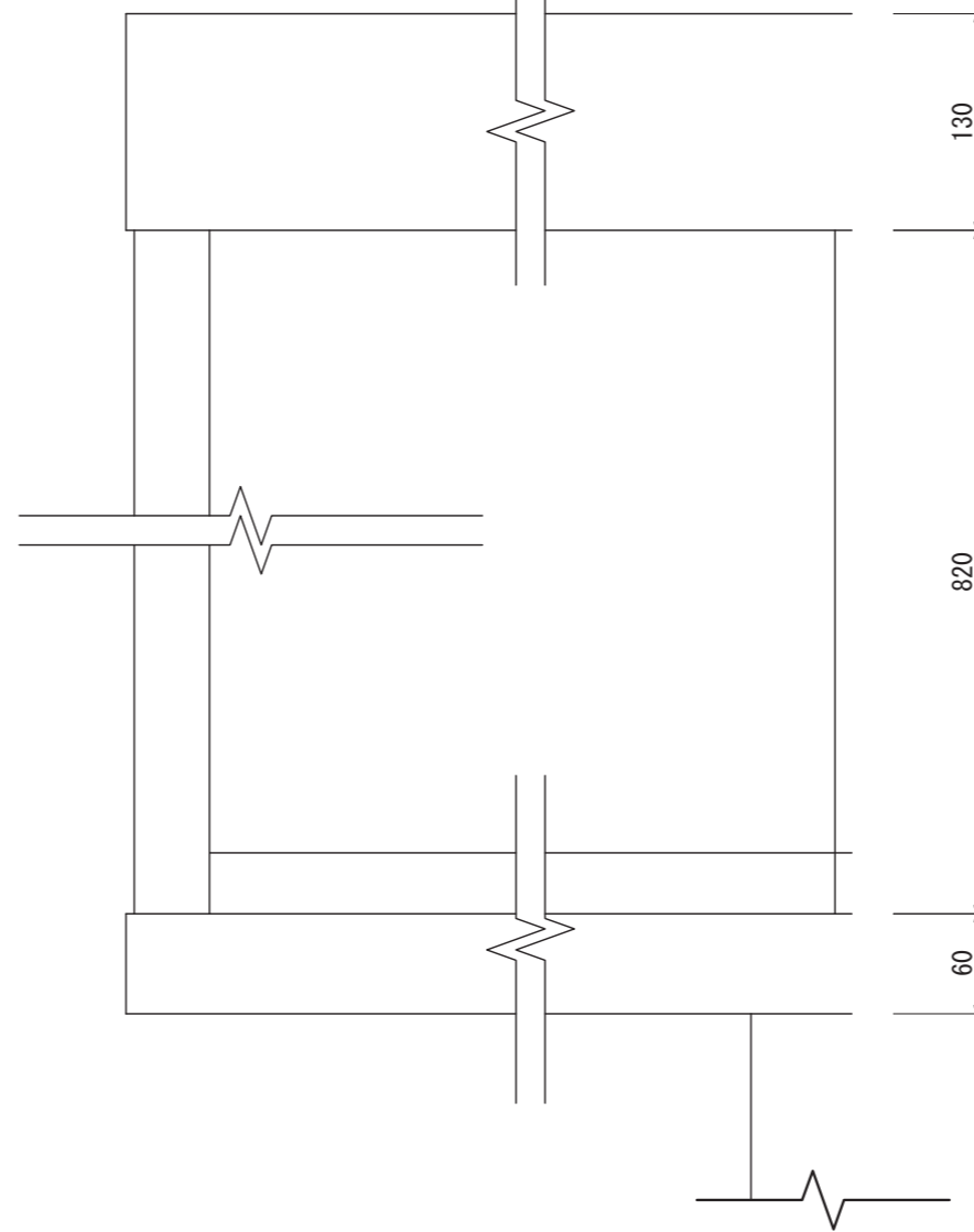
【正面図 S=1:5】
