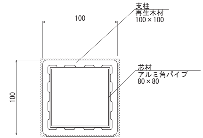
【断面図 S=1:3】
