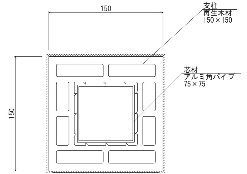
【断面図 S=1:3】
