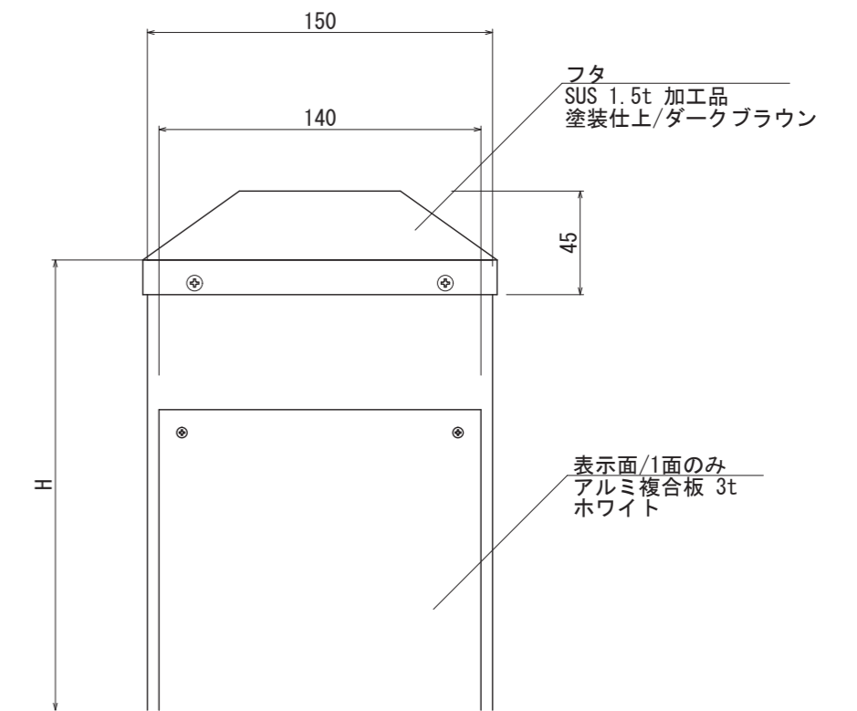
【正面図 S=1:3】
