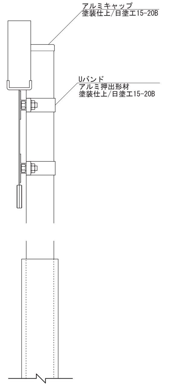
【側面図 S=1:5】
