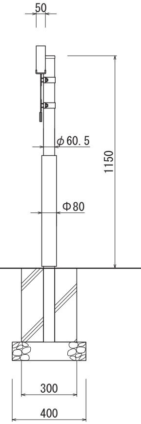
【側面図 S=1:20】
