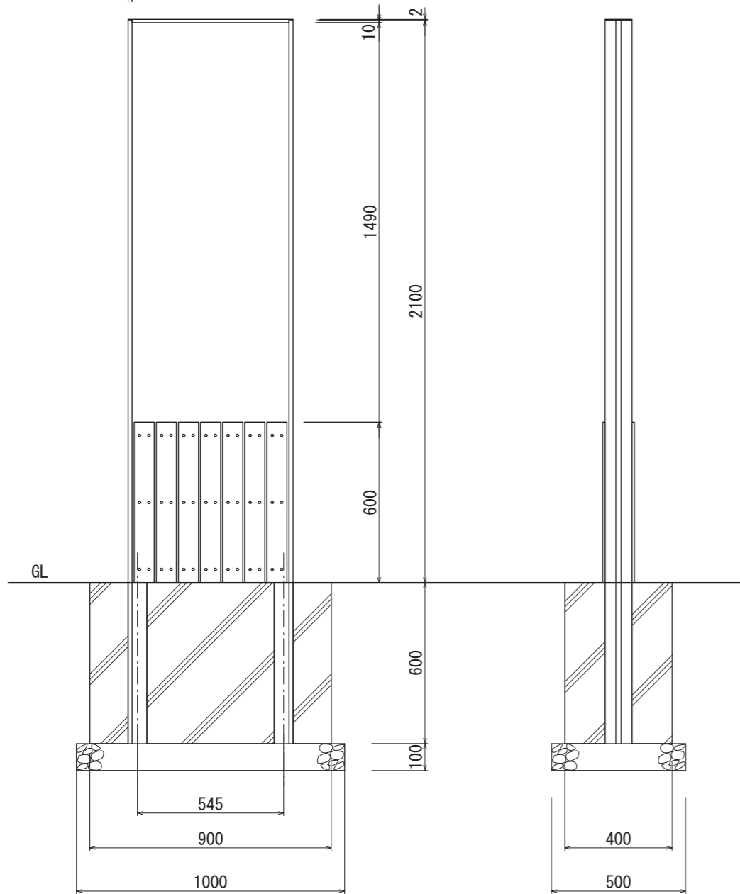
【正面図 S=1:20】
