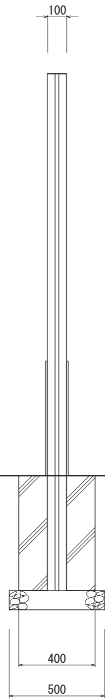
【側面図 S=1:20】
