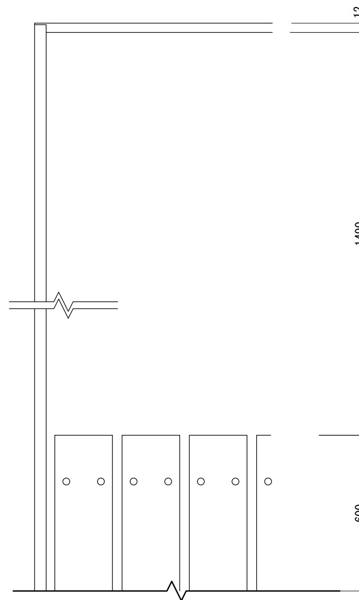
【正面図 S=1:5】
