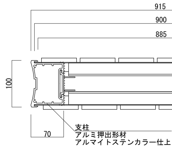
【平面図 S=1:5】
