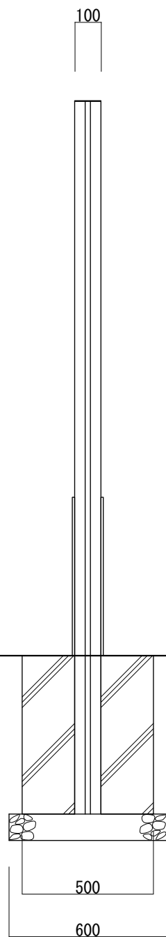
【側面図 S=1:20】
