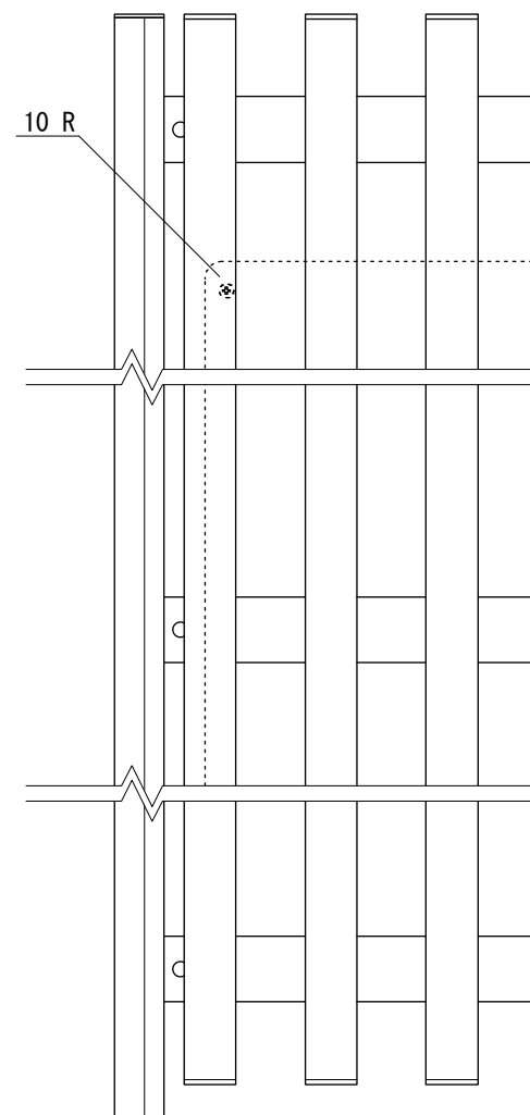
【正面図 S=1:5】
