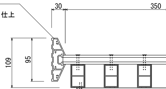
【平面図 S=1:5】
