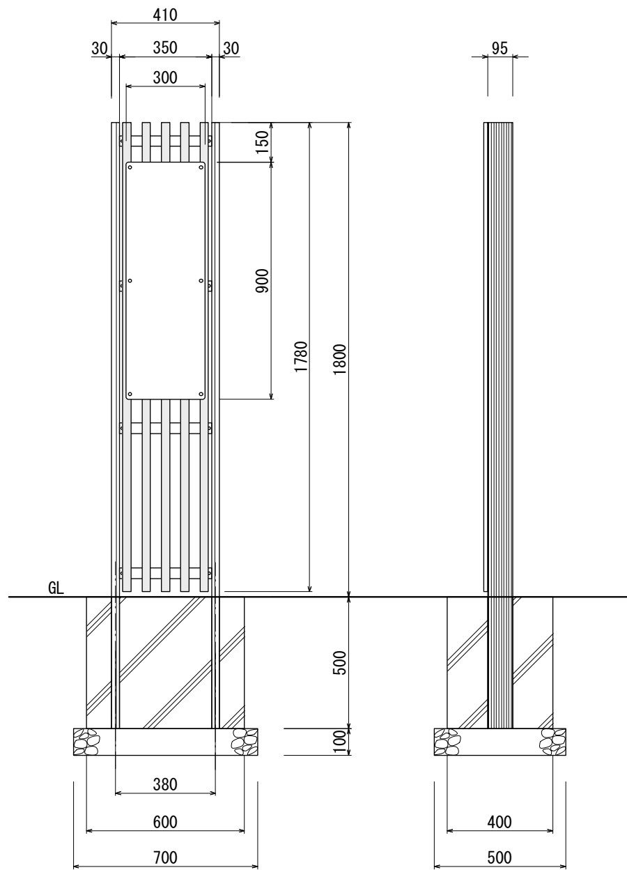
【正面図 S=1:20】
