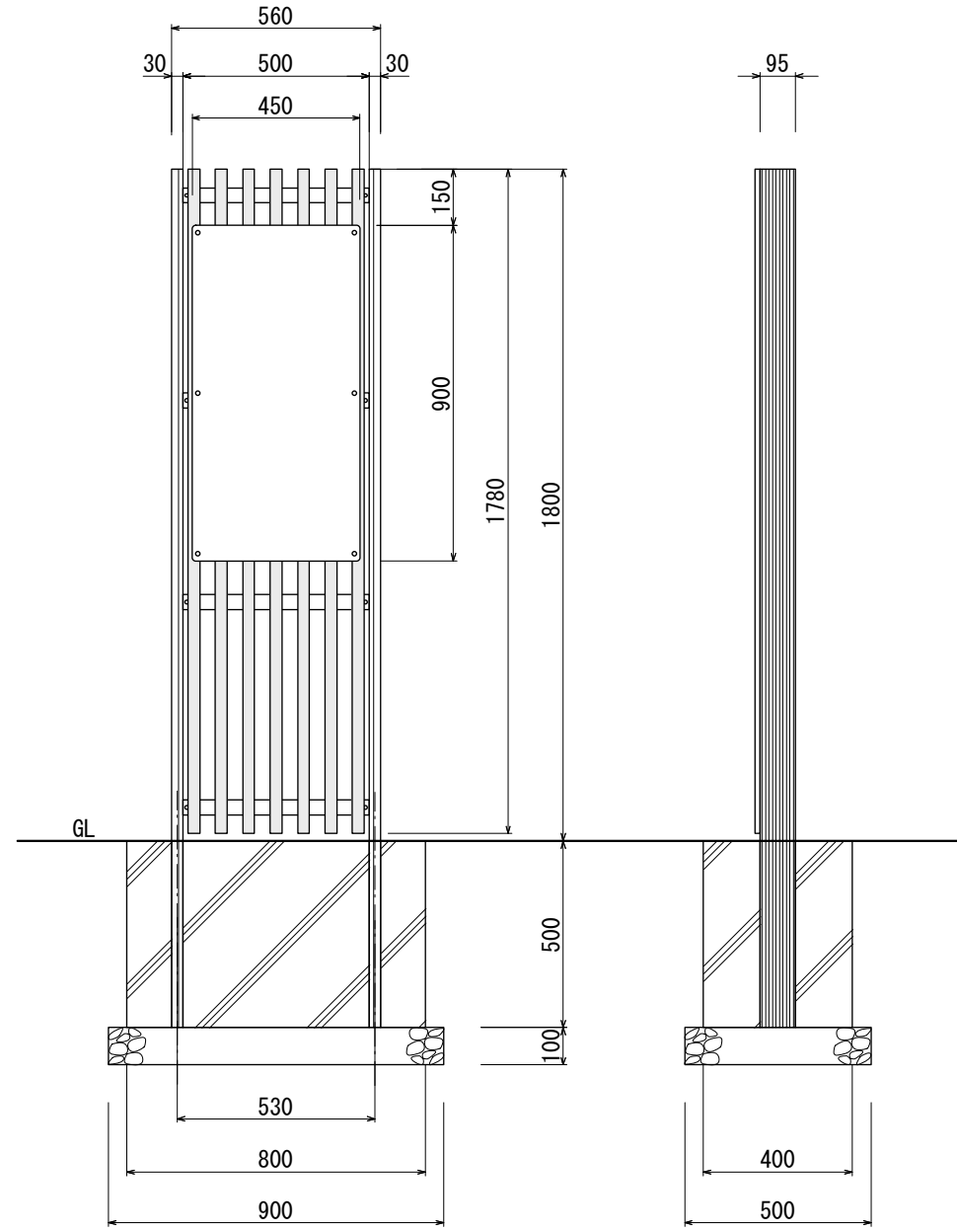
【正面図 S=1:20】
