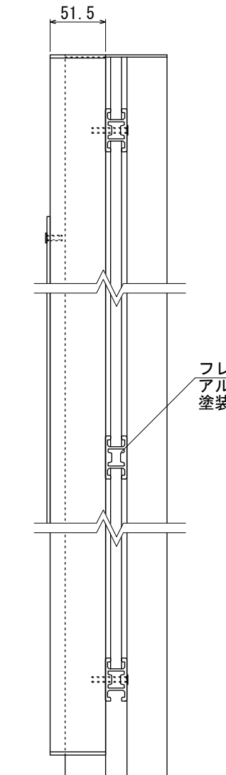
【側面図 S=1:5】
